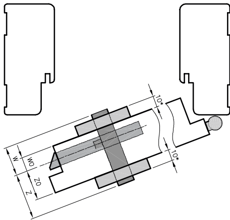
Dimensionering van de slotcilinder
