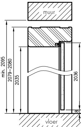
VERTICALE SECTIE OP VOOR GLAZEN DEUREN
