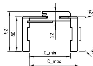
Doorsnede ORB 095-300
