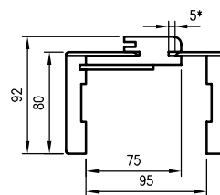
Doorsnede ORB 075
