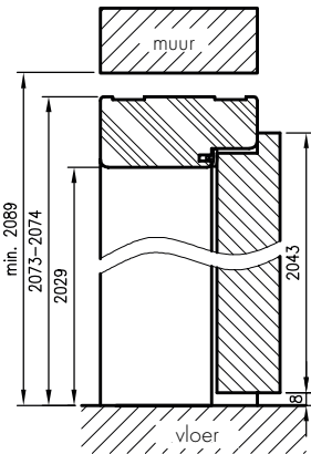
VERTICALE DOORSNEDE OP VOOR SPONNINGDEUREN
